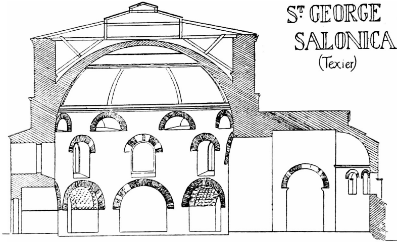
LONGITUDINAL SECTION
